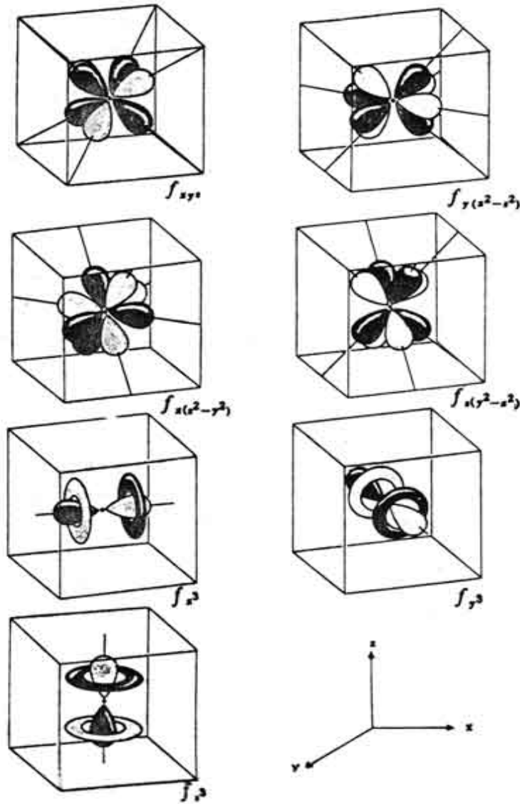
نمودار توابع موج زاویه‌ای هفت اوربیتال f
