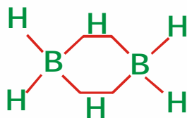
شکل (C): ساختار مولکول B_2H_6
