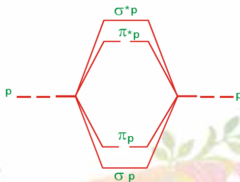
شکل: نمودار ترازهای انرژی برای ترکیب اوربیتال‌های p . از آنجا که اثر متقابل p (پیوند p ) ضعیف‌تر از اثر
